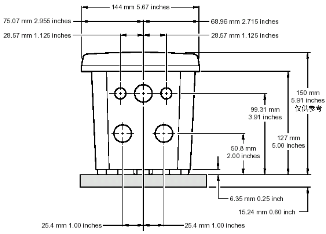
图 6 导线管开孔尺寸
