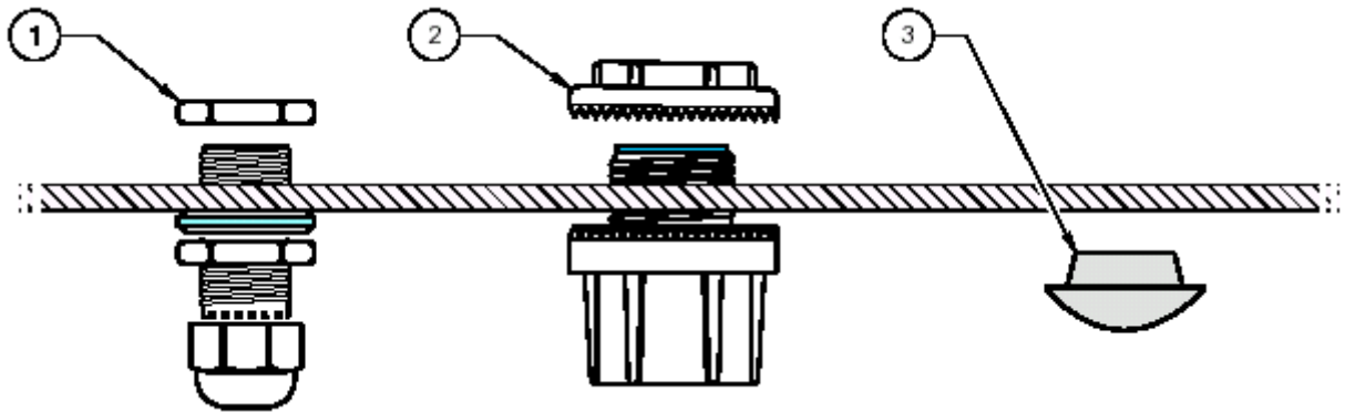
图 13 使用供选购的应变释放器及导线管密封塞
